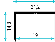
TD-2632 0,138 Kg/m U Çizgili Profil
