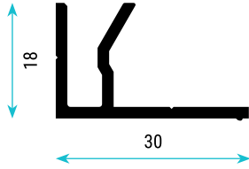
TD-3958 0,320 Kg/m F Profil Bitiş Profili
