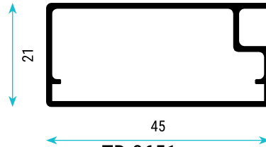
TD-3651 0,447 Kg/m Mobilya Kapak Geniş Çerçeve Profili
