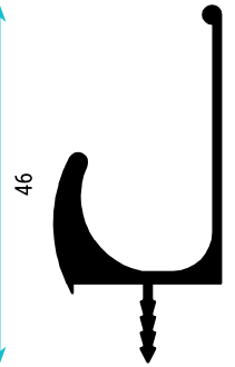
TD-3648 0,461 Kg/m Apaçi Kulp
