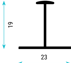
TD-3602 0,149 Kg/m 18mm Dar H Profili
