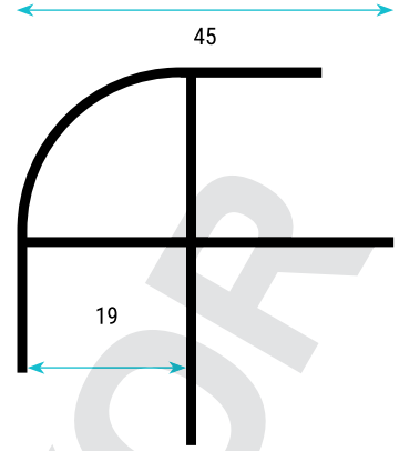
TD-2607 0,491 Kg/m Kolon Köşe Profili
