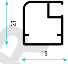
TD-3652 0,233 Kg/m Mobilya Kapak Dar Çerçeve Profili
