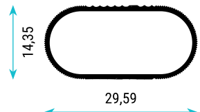
TD-989 0,178 Kg/m Büyük Oval Askı
