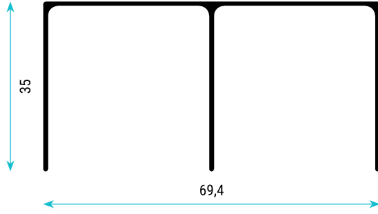
TD-976 0,447 Kg/m Üst Ray / Upper Rail
