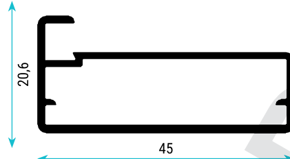
TD-3631 0,472 Kg/m Mobilya Kapak Geniş Çerçeve Profili
