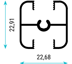
TD-979 0,244 Kg/m Orta Bağlantı Central Connect Profile
